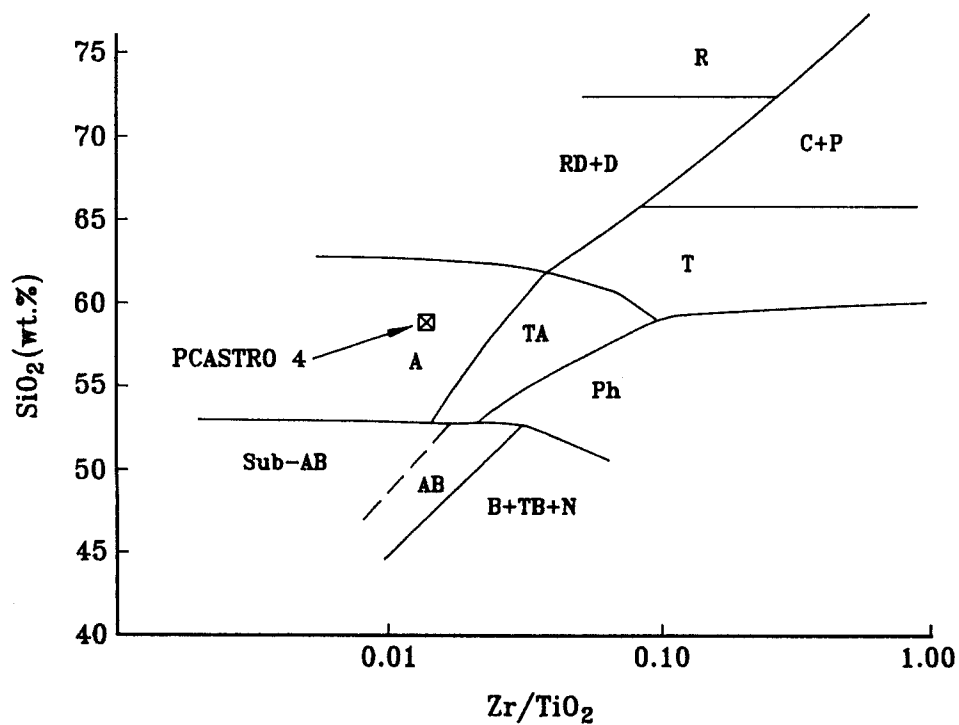
Fig. 7. Diagrama SiO_2 - Zr/TiO_2 de Floyd y Winchester (1978)
