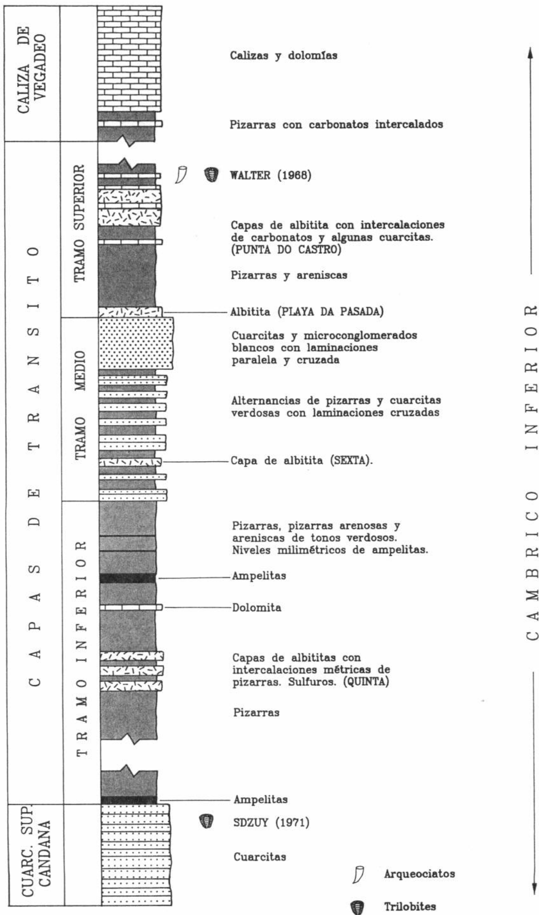
Fig. 8.- Columna estratigráfica esquemática de la parte superior del Grupo Cándana en el Distrito de Foz-Barreiros.
