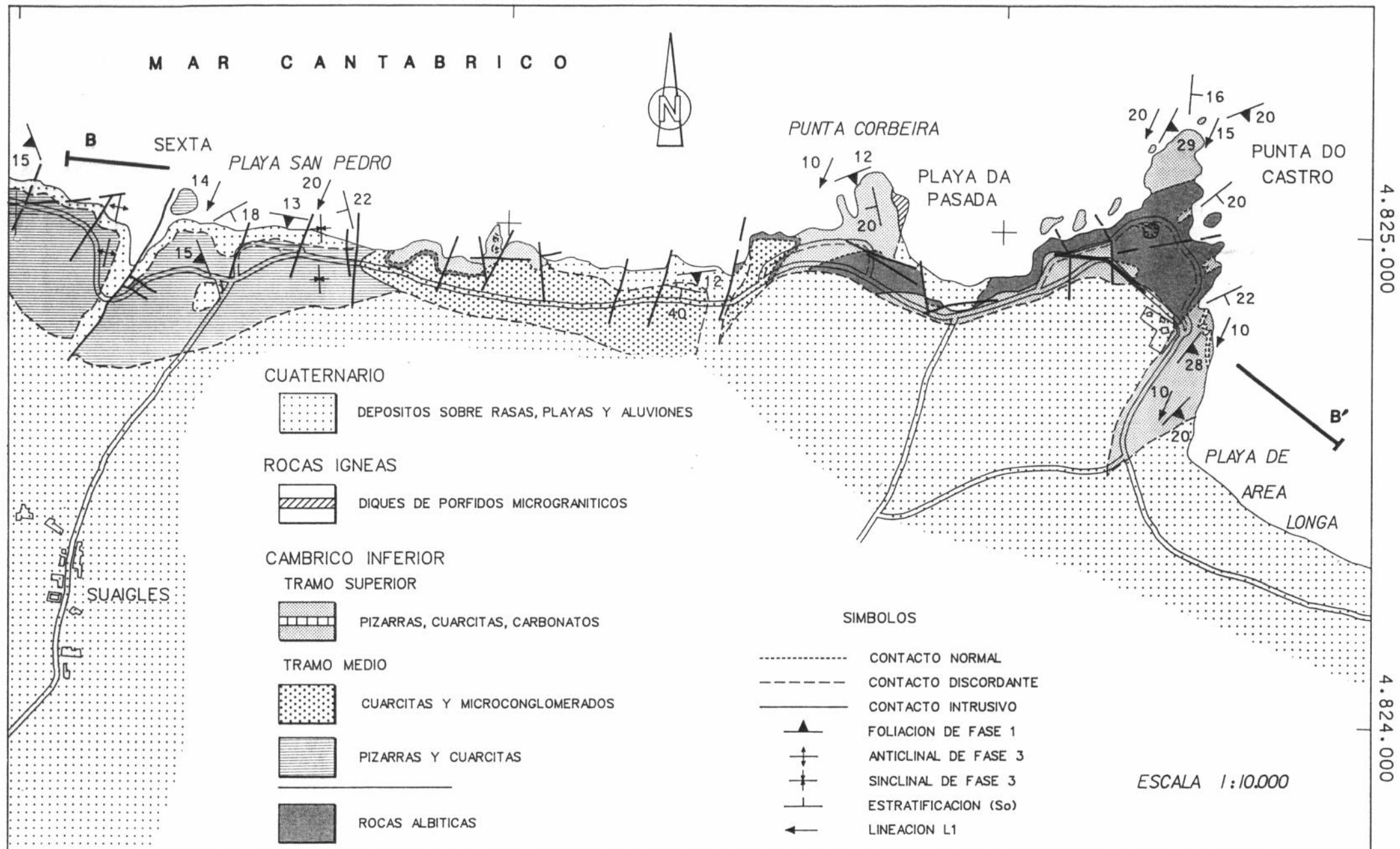
Fig. II. Mapa geológico de los Indicios Sexta y Playa da Pasada, y del yacimiento Punta do Castro.
