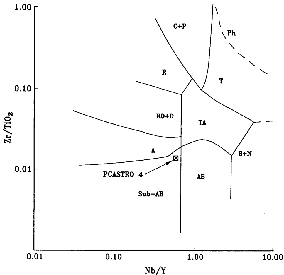
Fig. 6. Diagrama Zr/TiO_2 - Nb/Y de Floyd y Winchester (1978). Sub-AB: basaltos subalcalinos. AB: basaltos alcalinos, hawaitas, mugearitas, traquibasaltos. B+N: Basanitas y Nefelinitas. A: Andesitas. TA: Traquiandesitas. RD+D: Riodacitas y Dacitas. T: Traquitas. R: Riolitas. C+P: Comenditas y Panteleritas. Ph: Fonolitas.
