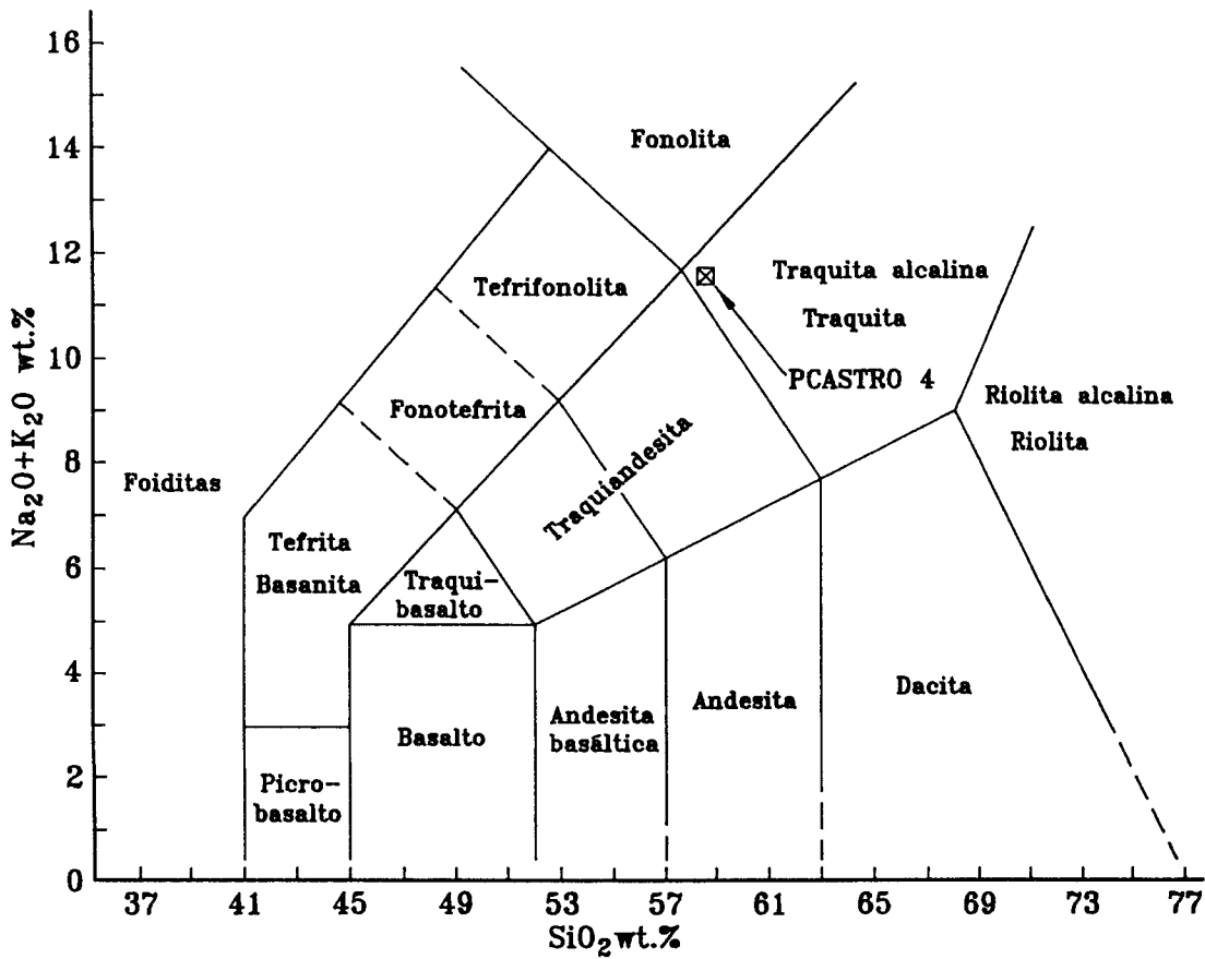
Fig. 5. Diagrama TAS. Proyección de la muestra PCastro 4. (Silice-álcalis).
