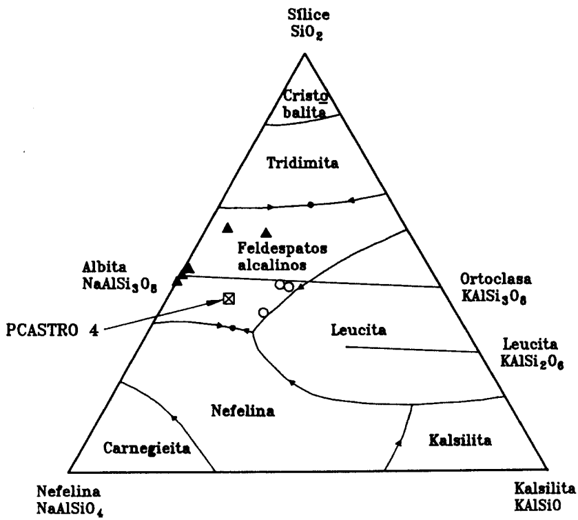
Fig 4. Diagrama Si-Ne-Ks. Proyección de la muestra PCastro 4. ○ Rocas volcánicas de Canarias. ▲ Rocas albiticas.
